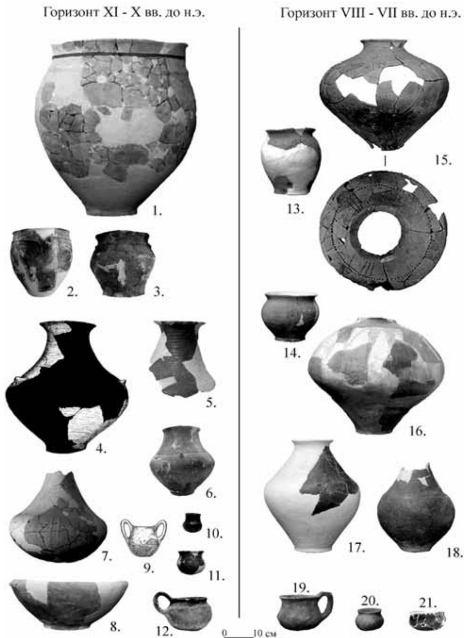
Рис. 1 / Fig. 1. Керамические комплексы финала поздней бронзы и начала раннего железа Предгорного Крыма: 1, 4, 7, 8, 9, 11, 12, 17, 19, 20 – пос. Уч-Баш [10]; 2, 3, 6, 10 – пос. Льговское-2017 [14] (кубок №10 – фото автора); 5, 12, 13, 14, 16, 18 – пос. Сахарная головка [10]; 15 – пос. Фронтное 2 [14]; 21 – пам. Пролом 1 [9] / Ceramic complexes of the final of the Late Bronze Age and the beginning of the Early Iron of the Foothill Crimea: 1, 4, 7, 8, 9, 11, 12, 17, 19, 20 – Uch-Bash; 2, 3, 6, 10, - Lgovskoe; 5, 12, 13, 14, 16, 18 – Saharnaya Golovka; 15 – Frontovoe 2; 21 – Prolom 1 1
